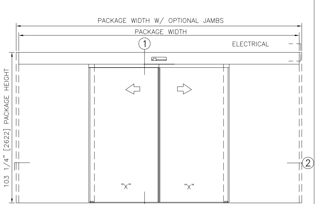
ELEVATION
