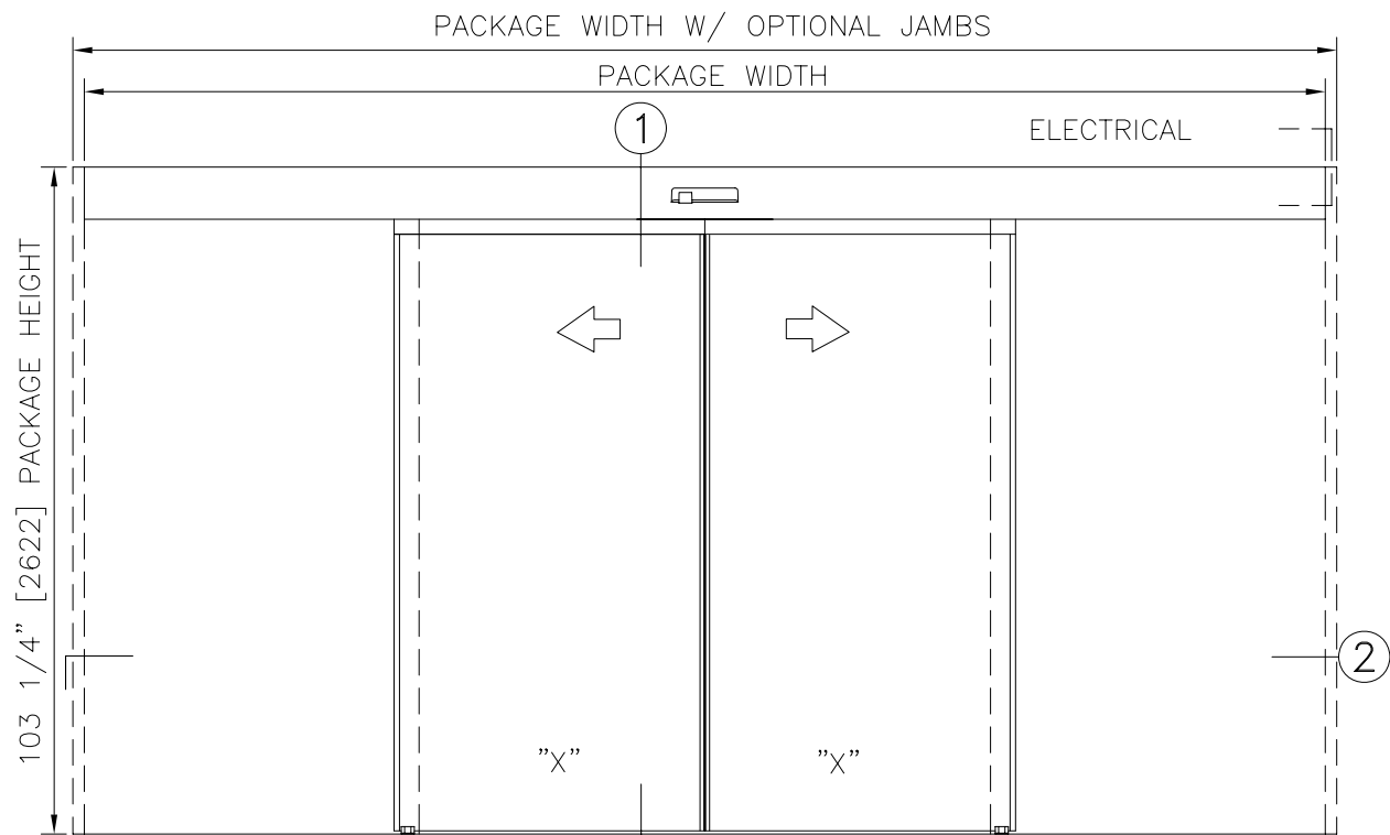
ELEVATION VIEW SCALE: 3/8" = 1'-0"
