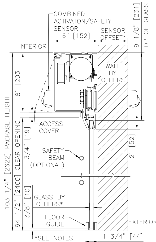
① VERTICAL SECTION SCALE: 2" = 1'-0"
