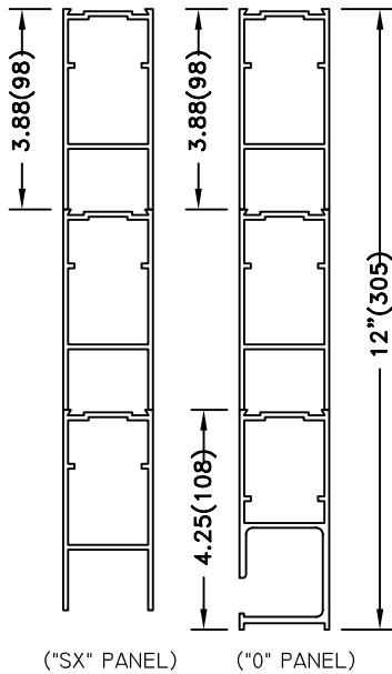
12"
