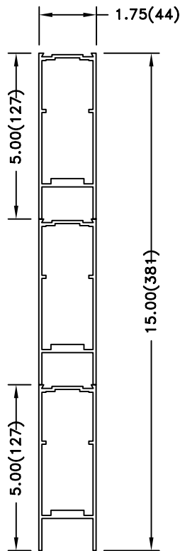
15"
